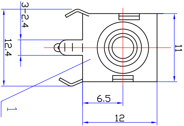
印制线路板推荐开孔尺寸 由下向上插
