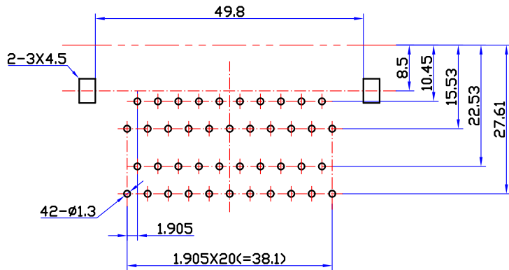
印制线路板推荐开孔尺寸
