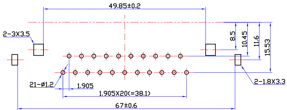
印制电路板推荐开孔尺寸
