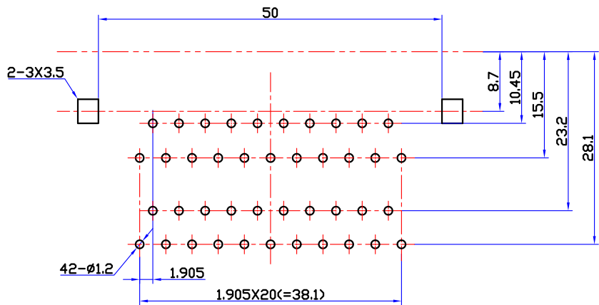
印制电路板推荐开孔尺寸
