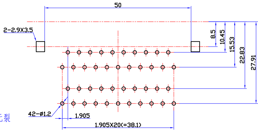
印制线路板推荐开孔尺寸
