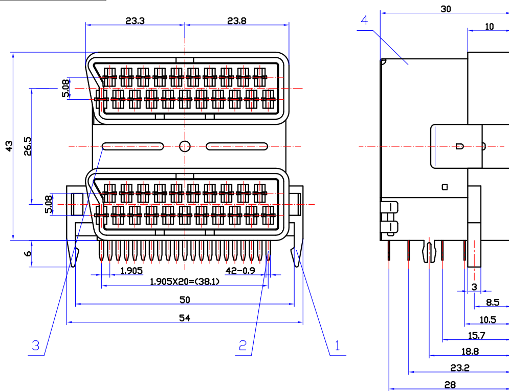
印制线路板推荐开孔尺寸
