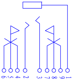
接点示意图
