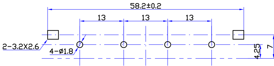
印制线路板推荐开孔尺寸
