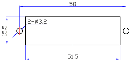
安装板推荐开孔尺寸
