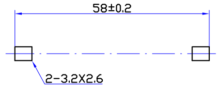
印制线路板推荐开孔尺寸
