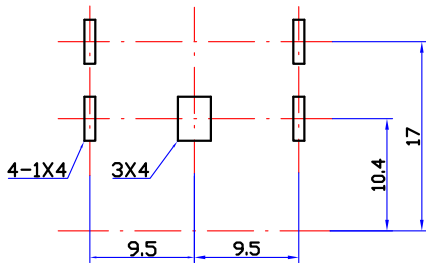
印制线路板推荐开孔尺寸
