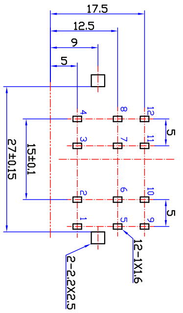
印制线路板推荐开孔尺寸 从向上下插 ⊗
