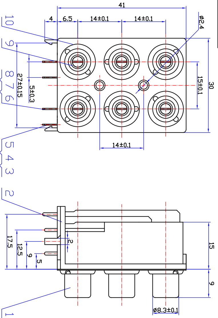
接点示意图
