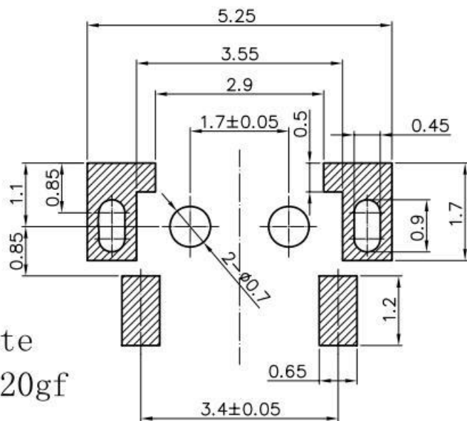
PCB. 焊接尺寸图
