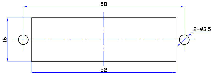
安装板推荐开孔尺寸
