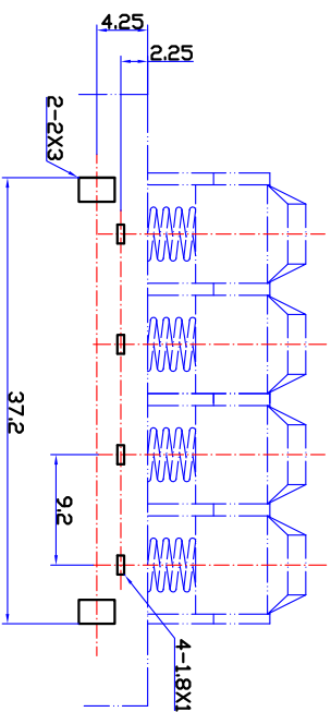
印制线路板推荐开孔尺寸
