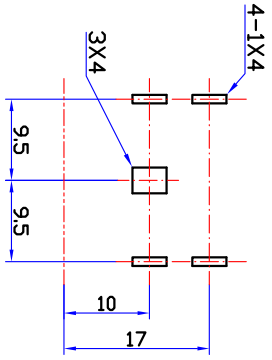
印制线路板推荐开孔尺寸
