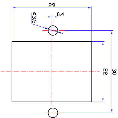
安装板推荐开孔尺寸
